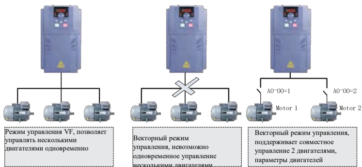
Рисунок 4-26 Переключение нескольких комплектов двигателей
