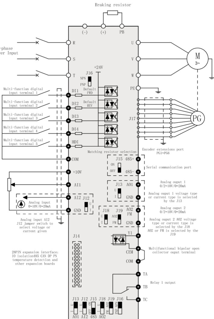
Рисунок 3-7 (4T/7T) Трехфазный инвертор мощностью более 4,0 кВт
