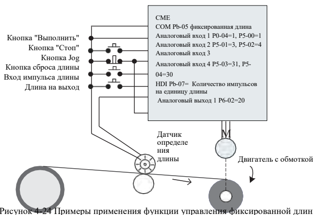
Рисунок 4-24 Примеры применения функции управления фиксированной длины
