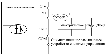
Рисунок 3-15 Схема подключения клеммы цифрового выхода Y1
