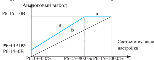
Рисунок 4-29 Принципиальная схема Аналоговый выход
