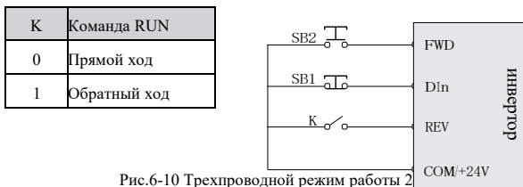
Рис.6-10 Трехпроводной режим работы 2
