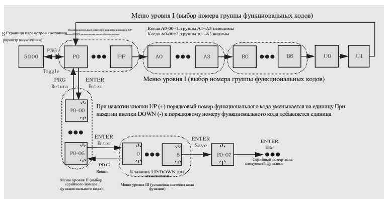
Рисунок 4-2 Блок-схема работы трехуровневого меню
