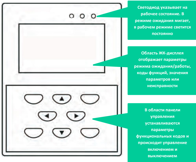
Рисунок 2-1 Панель управления
