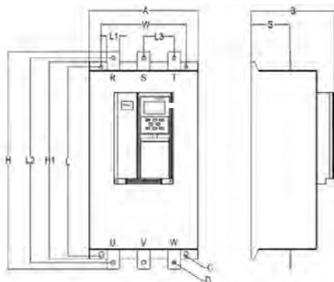
Рис. 6-1. Габаритные и установочные размеры корпуса и медных шин для кода RR2, RR3.
